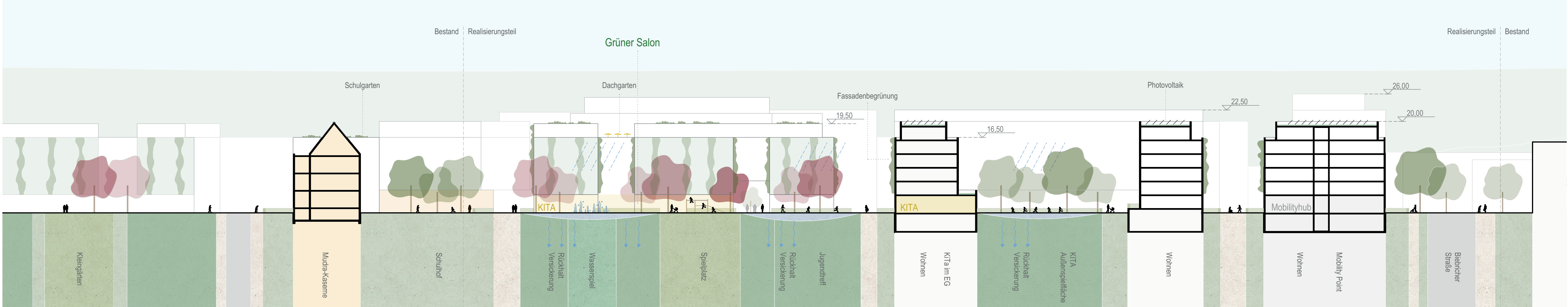
SYSTEMSCHNITT A-A 1:500
