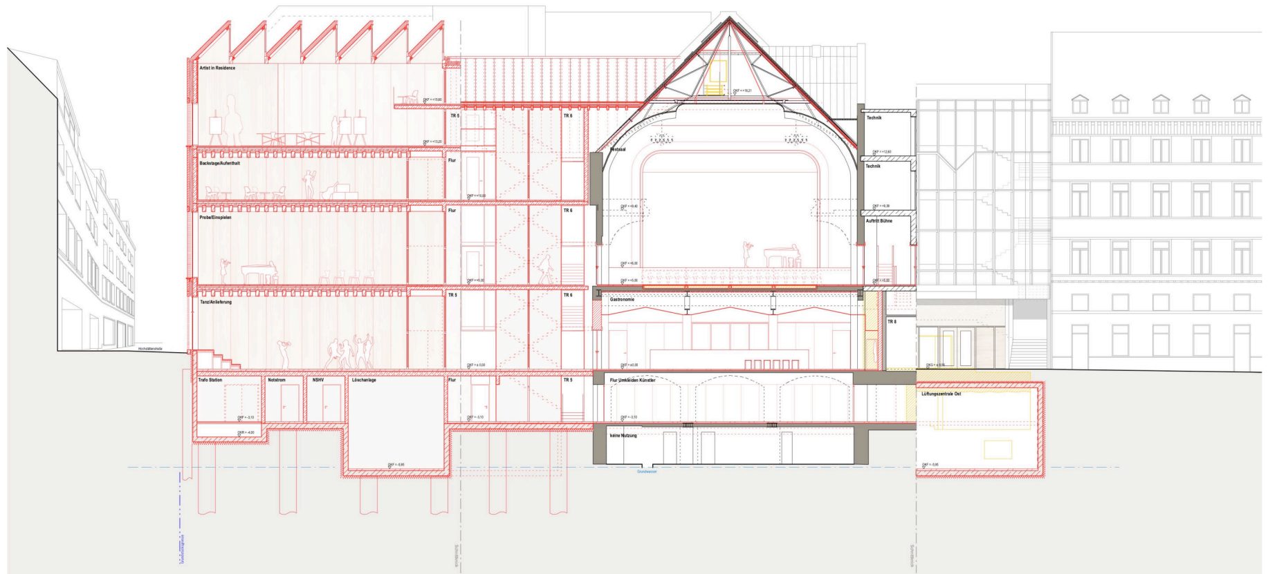
Querschnitt Wiesbaden: Walhalla
