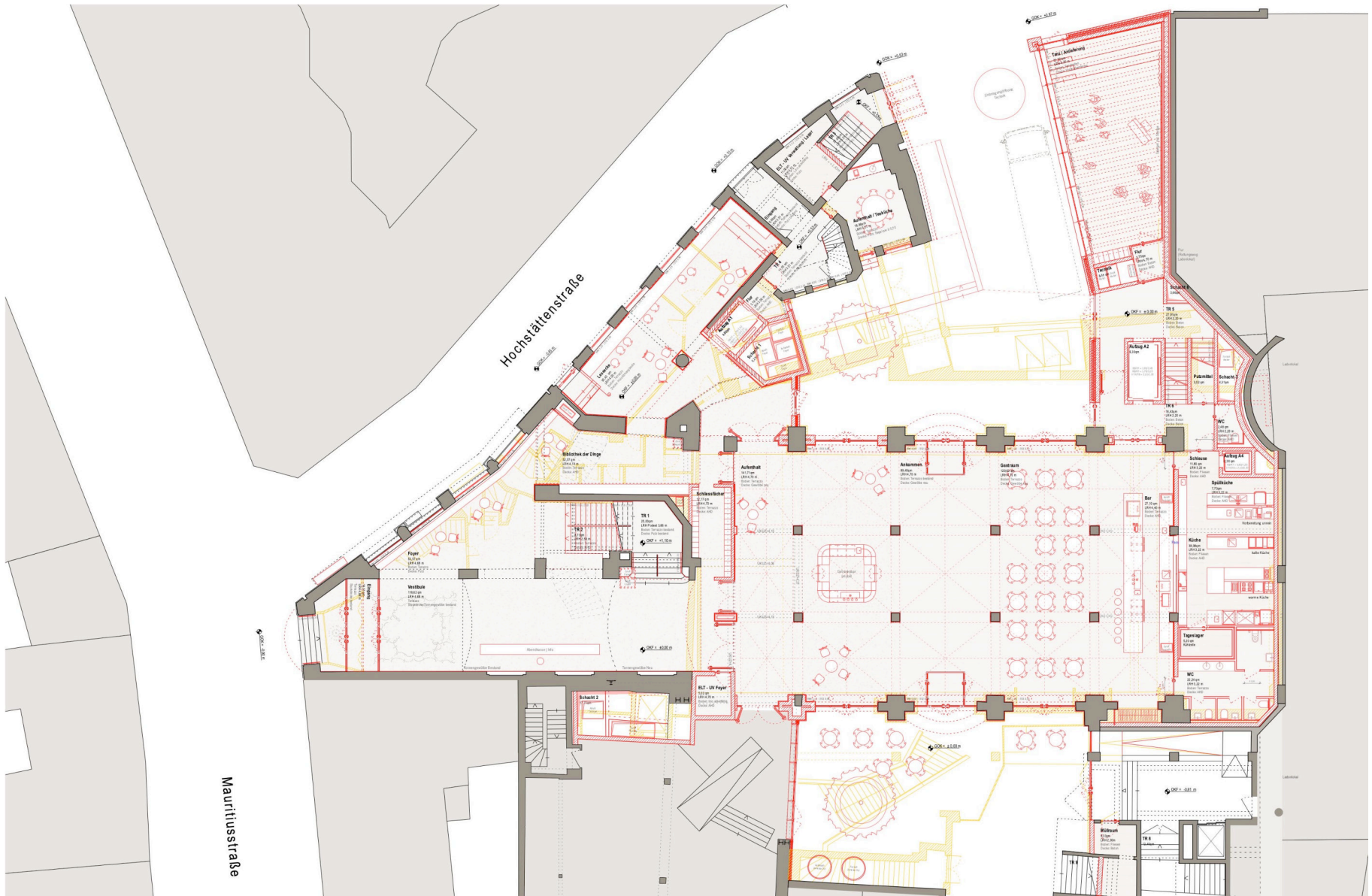
Grundriss 00.EG Wiesbaden: Walhalla
