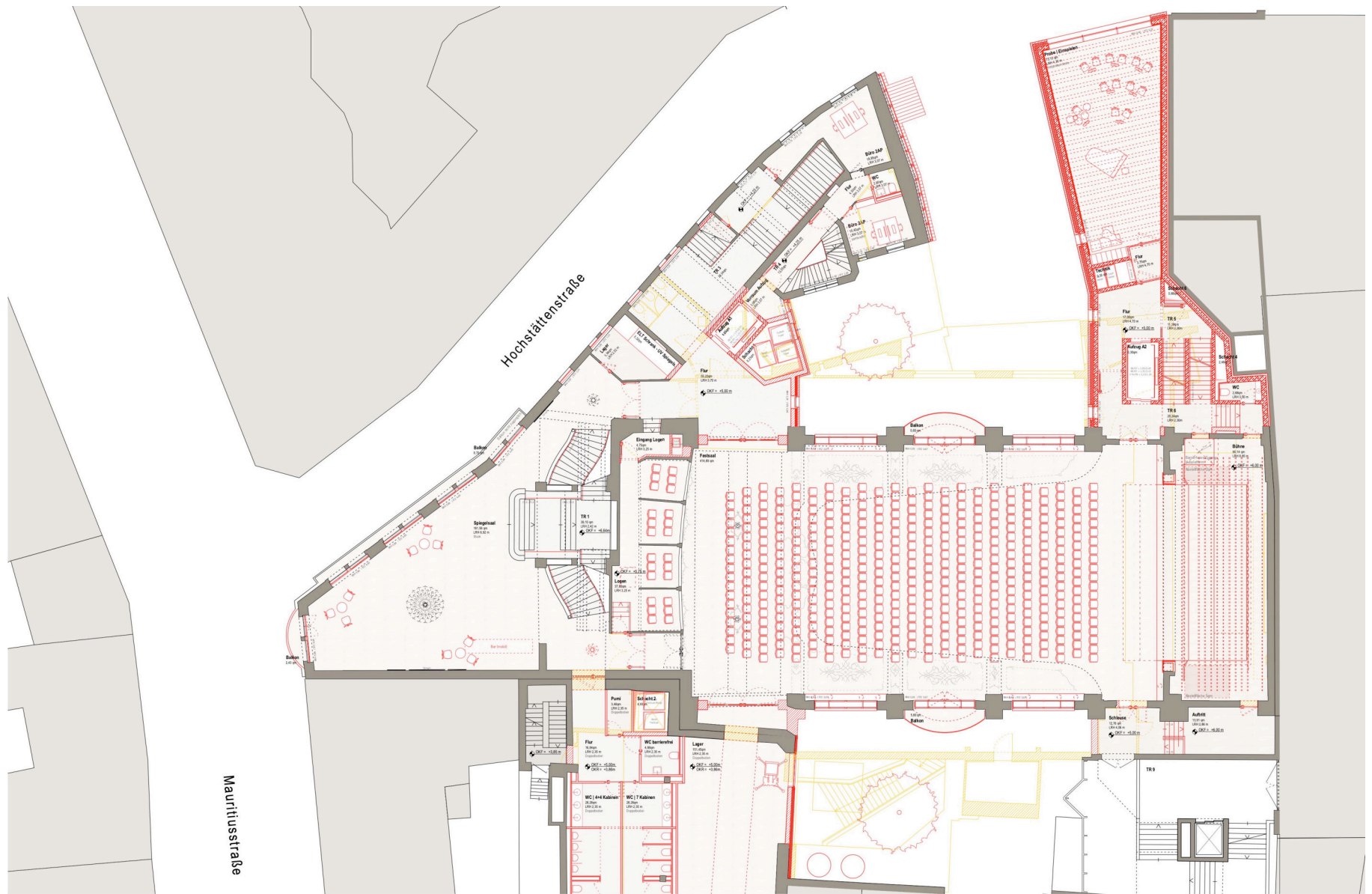
Grundriss 01.OG Wiesbaden: Walhalla
