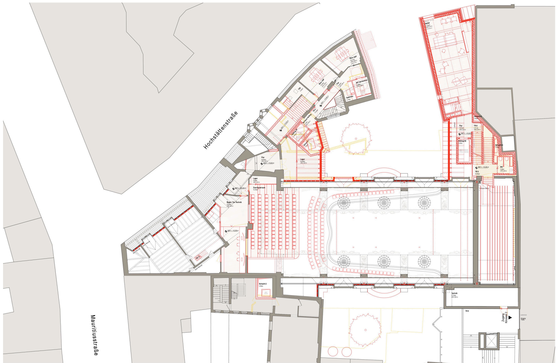
Grundriss 03.OG Wiesbaden: Walhalla
