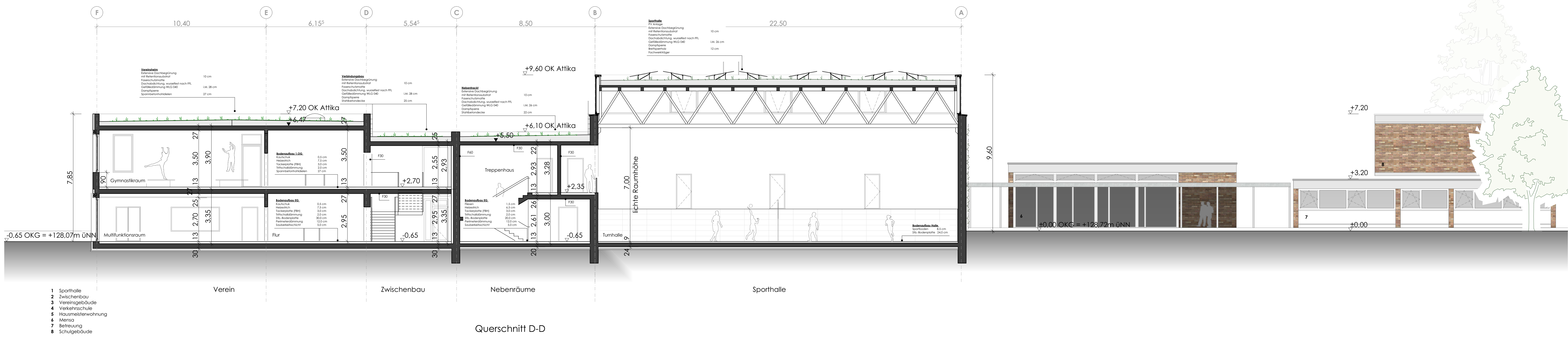
Querschnitt D-D
