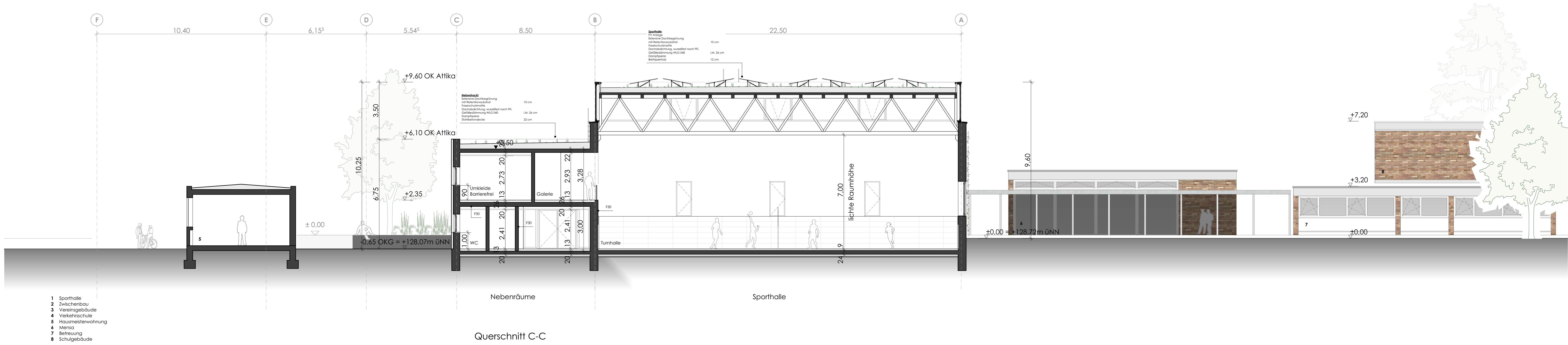
Querschnitt C-C
