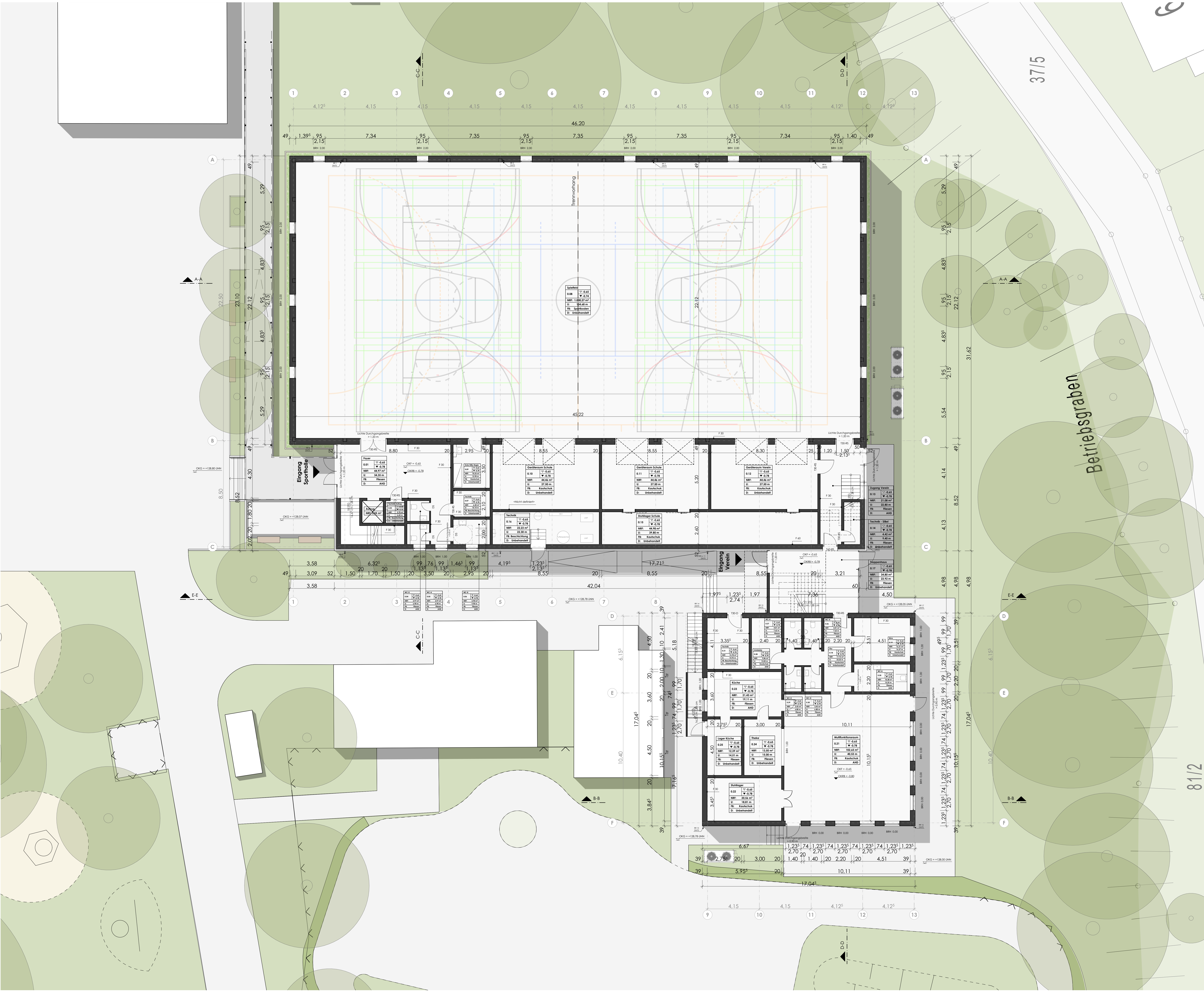
Grundriss Erdgeschoss
