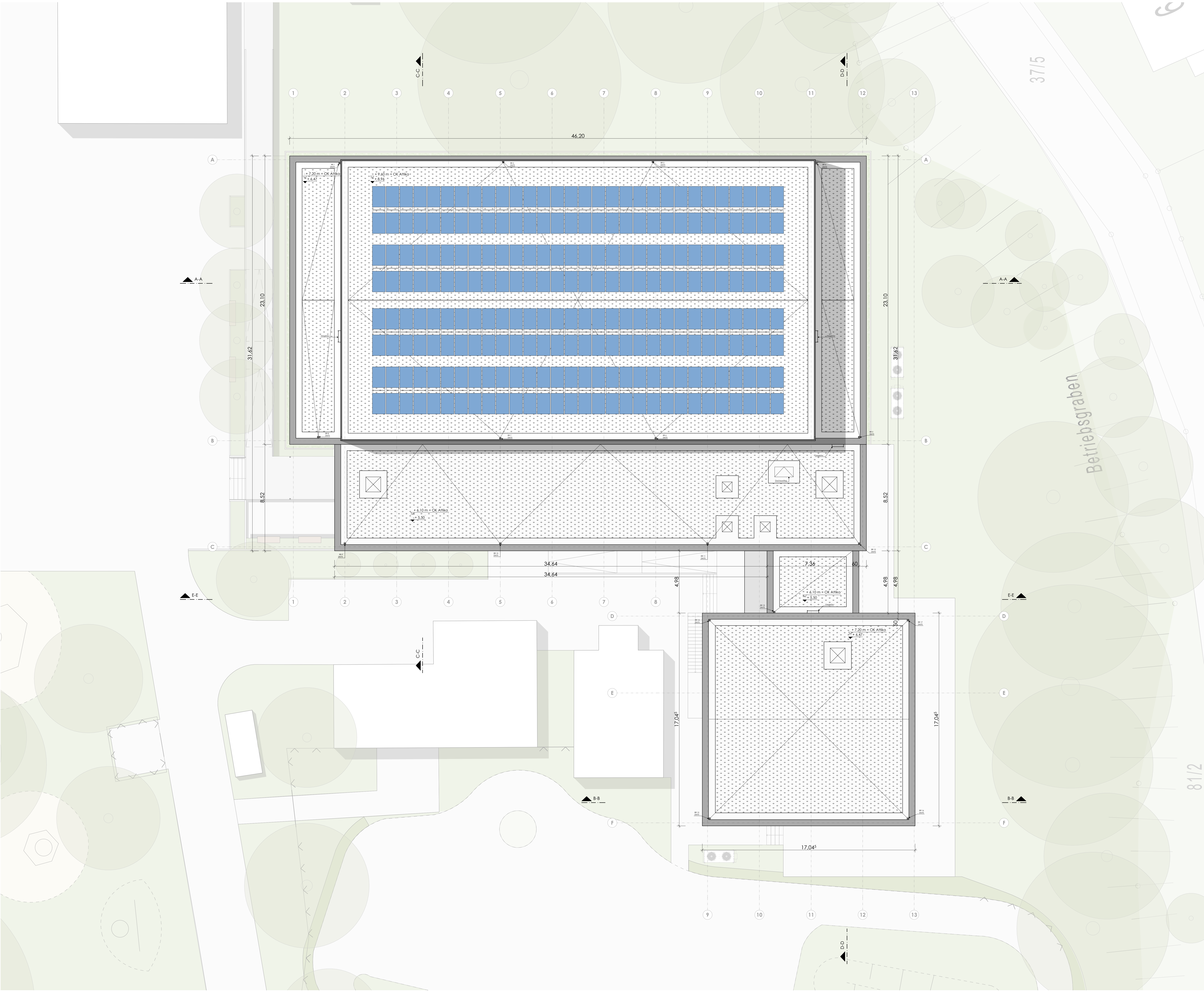
Dachaufsicht
