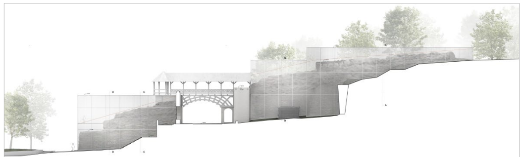
Ansicht Nord
