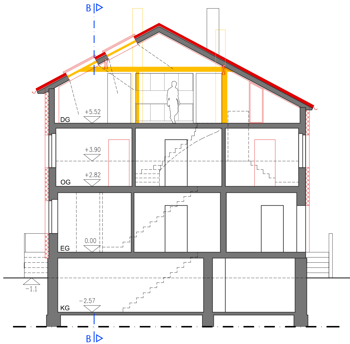
SCHNITT A
