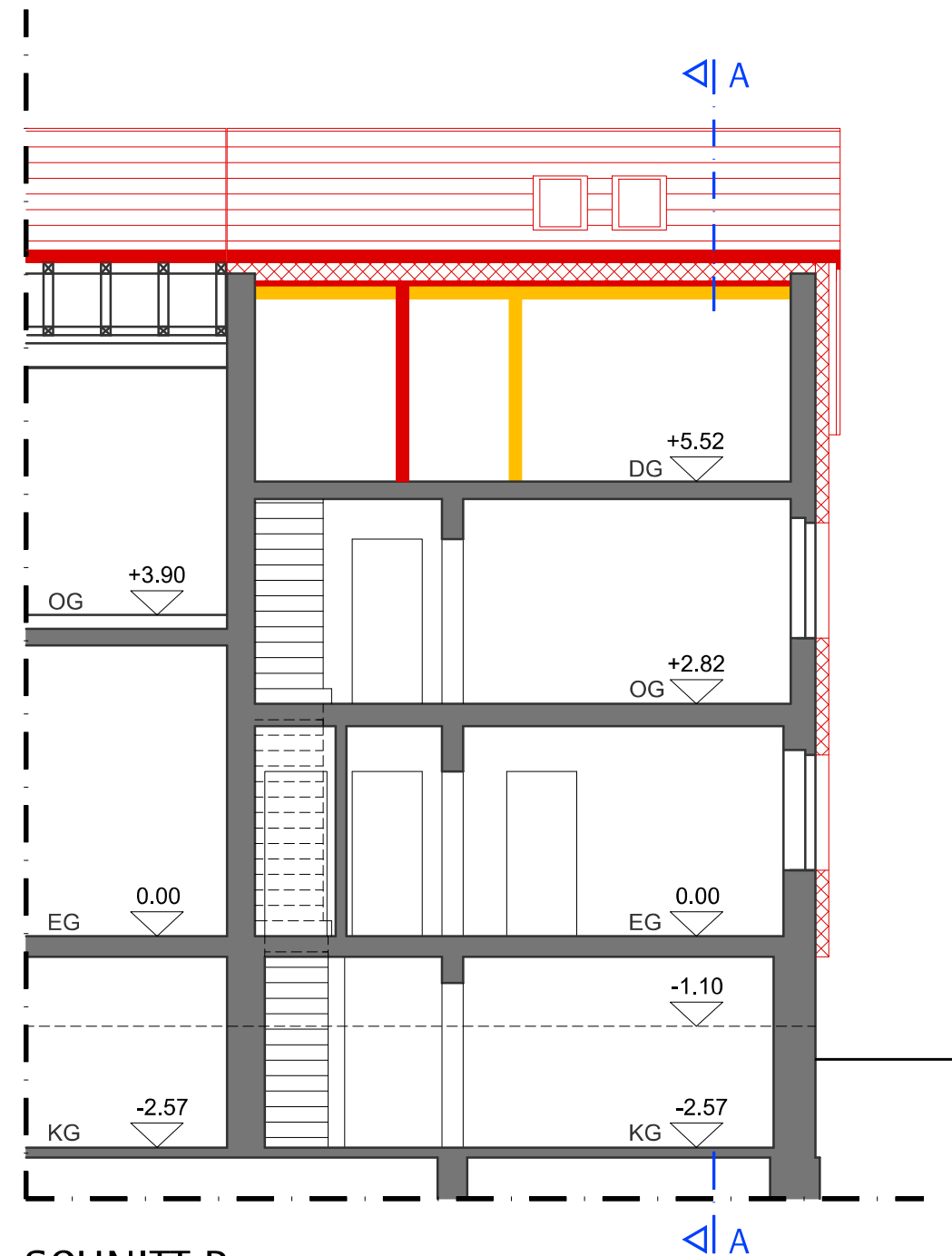
SCHNITT B
