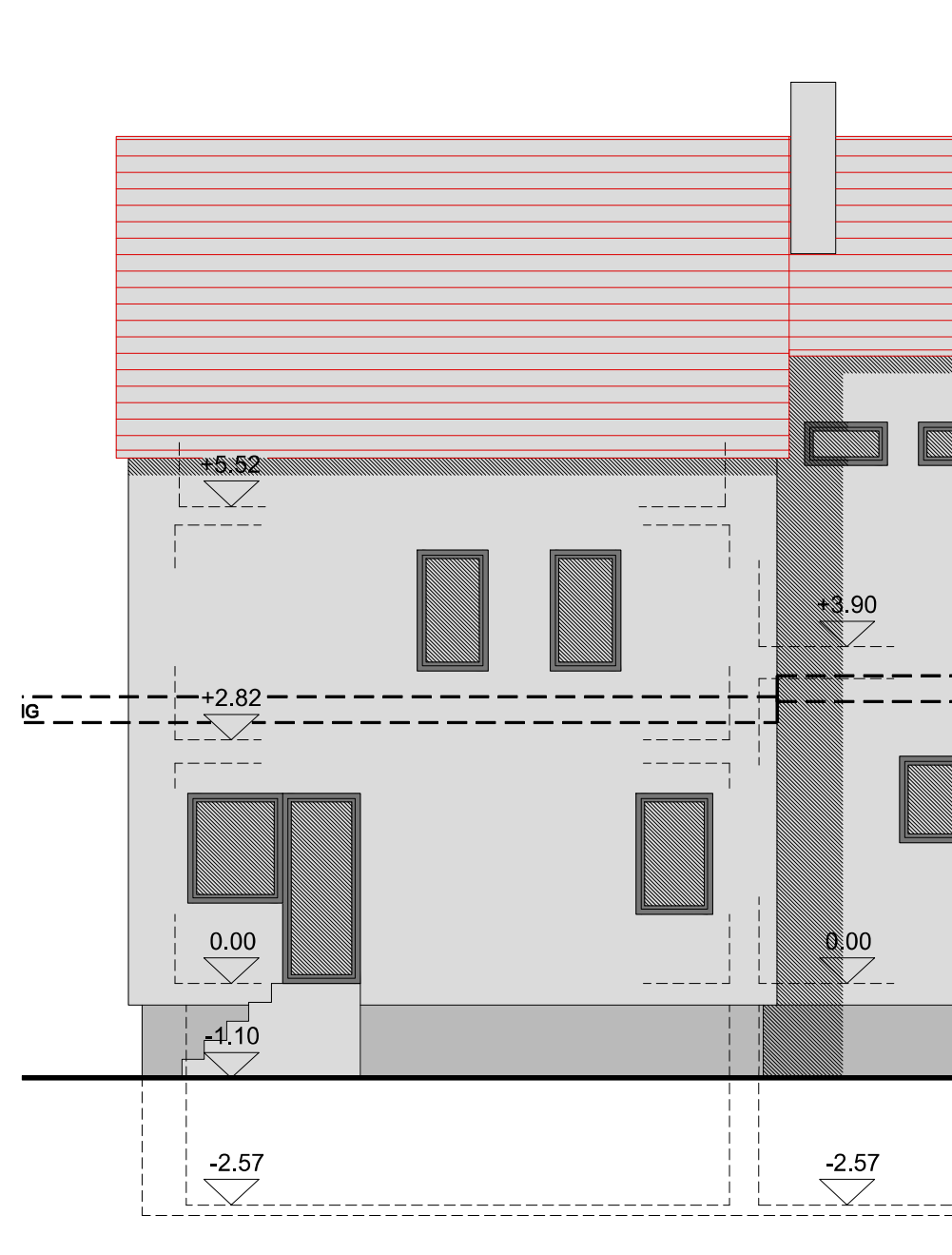
ANSICHT OST
