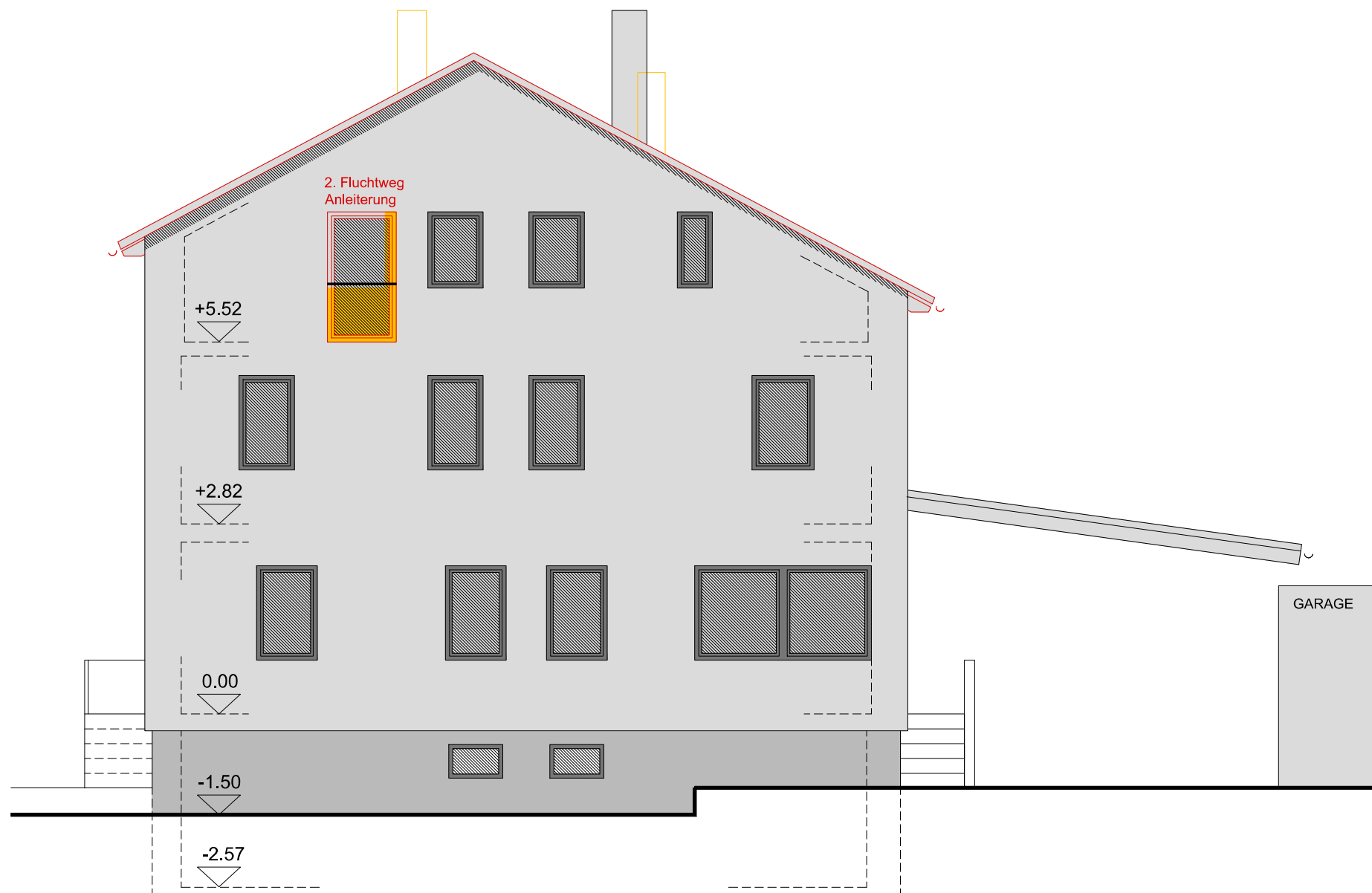
ANSICHT SÜD
