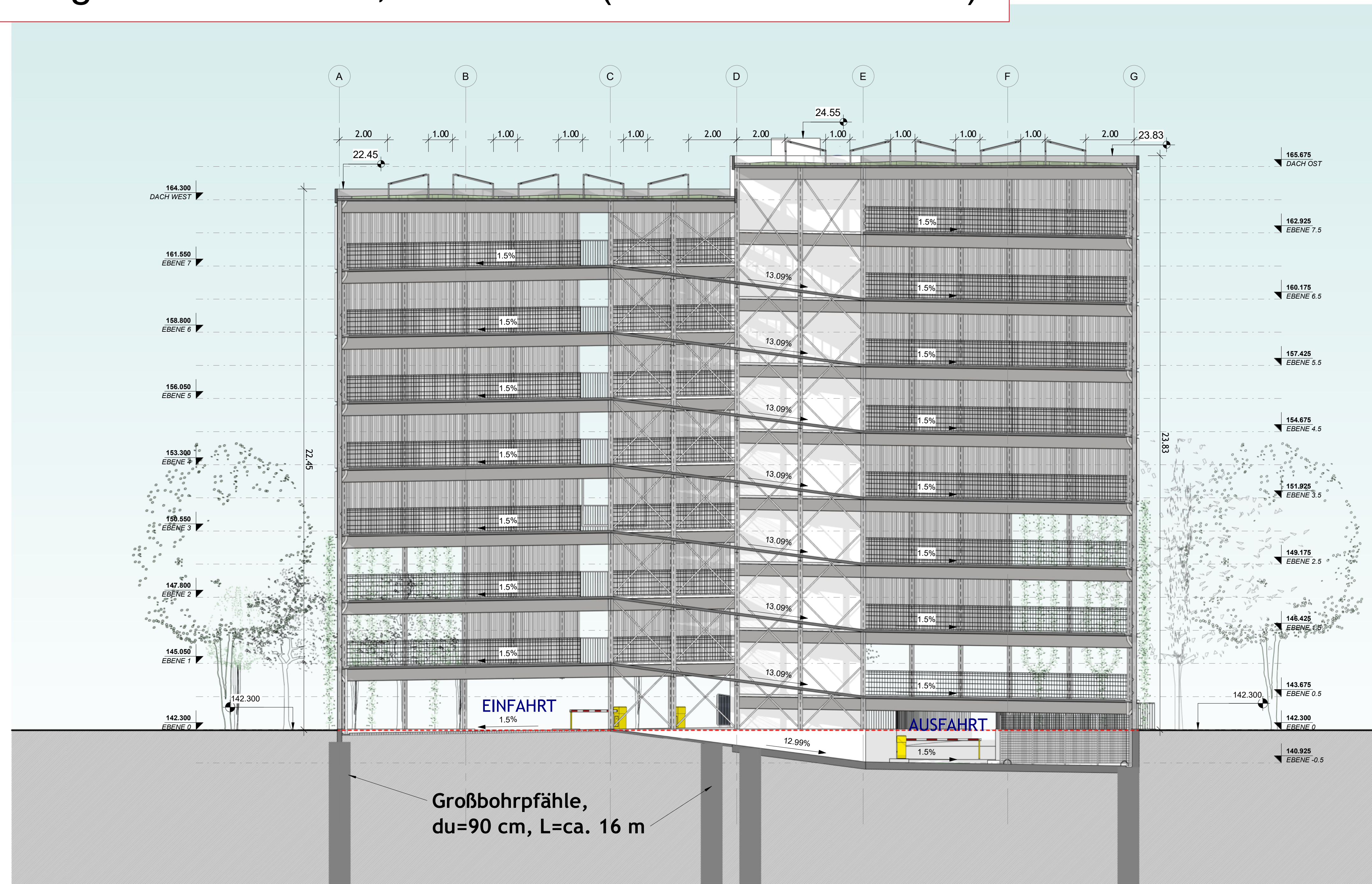
1 SCHNITT_AA 1 : 100
