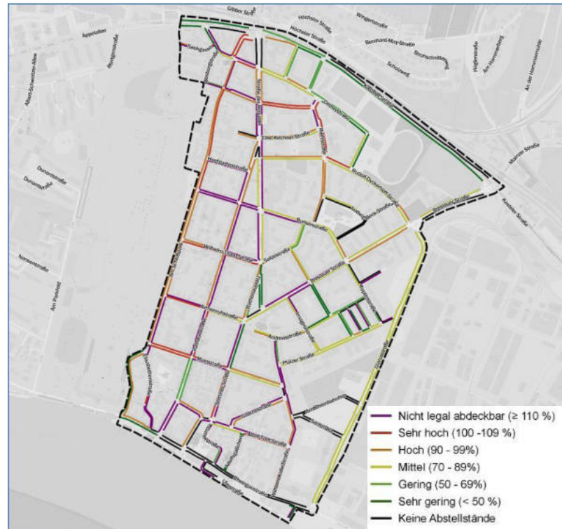
Abbildung 47: Beispiel zur Darstellung des Parkraumbelastungsgrads im öffentlichen Straßenraum
