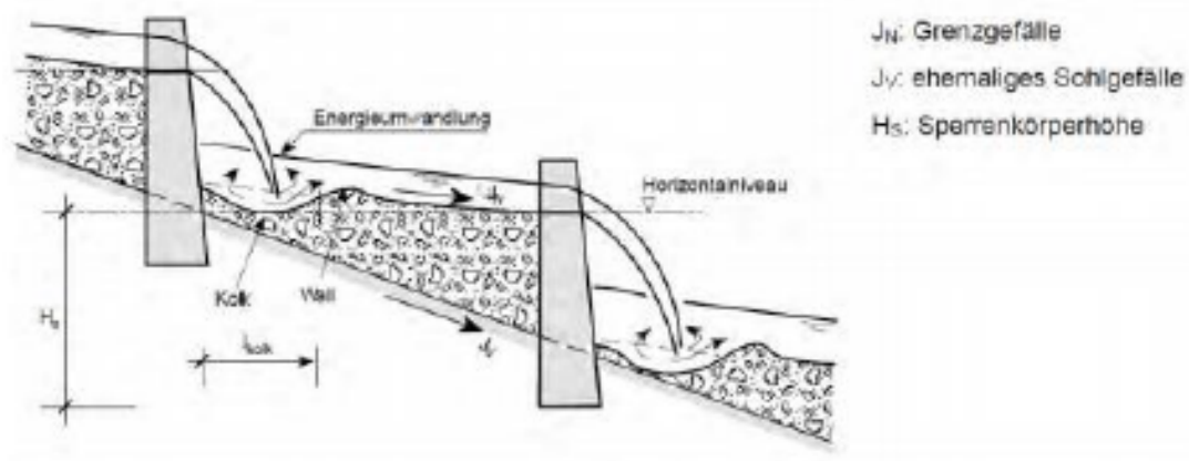
Abbildung 6: Schematische Darstellung im Längsprofil der Kolkbildung unterhalb von Sperrentreppen. (Quelle: Bergmeister et al. 2009, nach Böll 1997).
