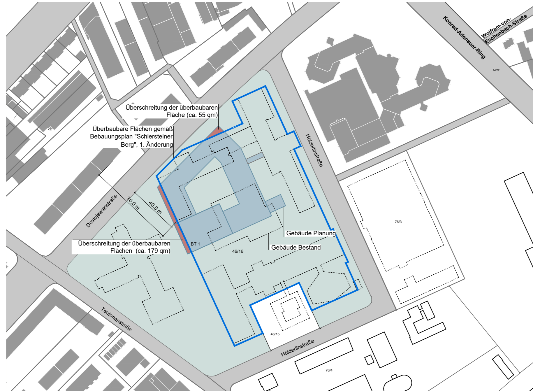
Abbildung 1: Überbaubare Grundstücksflächen
