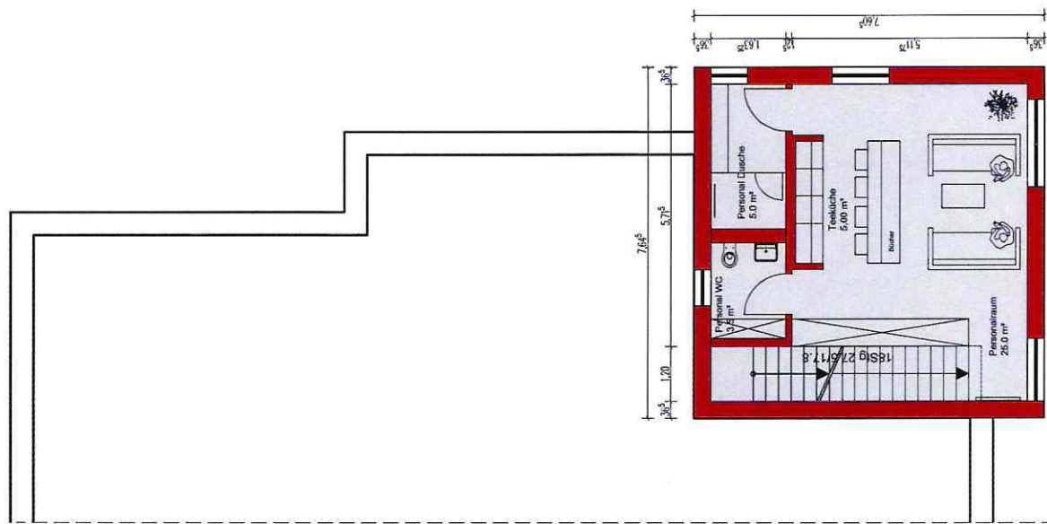
1. Obergeschoss
