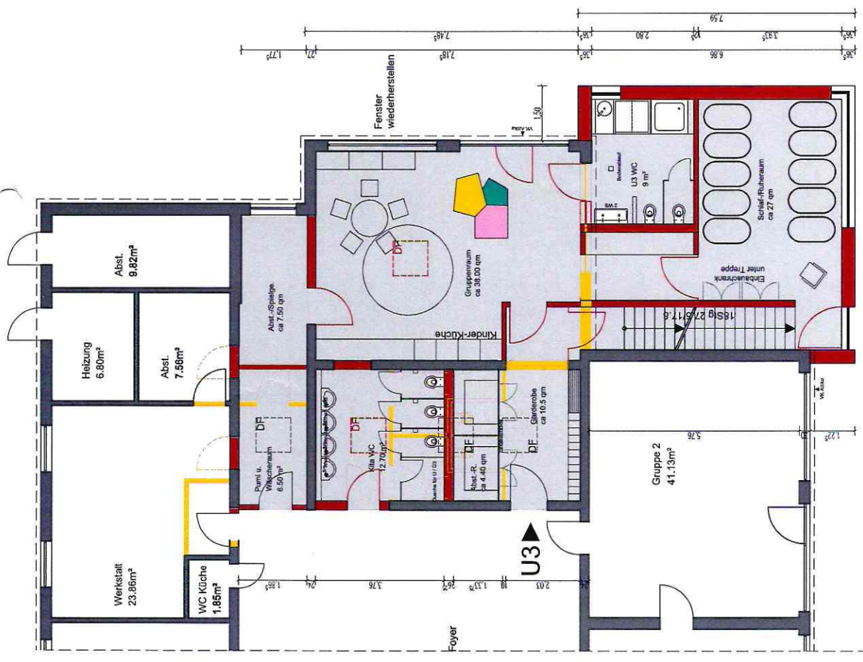
Erdgeschoss
