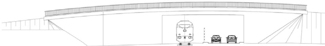
Abbildung: Geplante Brücke über die Ländchesbahn (Vorentwurf, Schnitt) Daten zur Brücke: lichte Höhe: 4,90 m; lichte Weite: 14,10 m Quelle: KREBS+KIEFER, Darmstadt, März 2014
