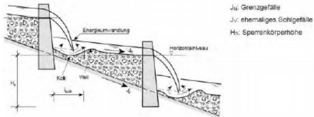
Abbildung 6: Schematische Darstellung im Längsprofil der Kolkbildung unterhalb von Sperrentreppen. (Quelle: Bergmeister et al. 2009, nach Böll 1997).
